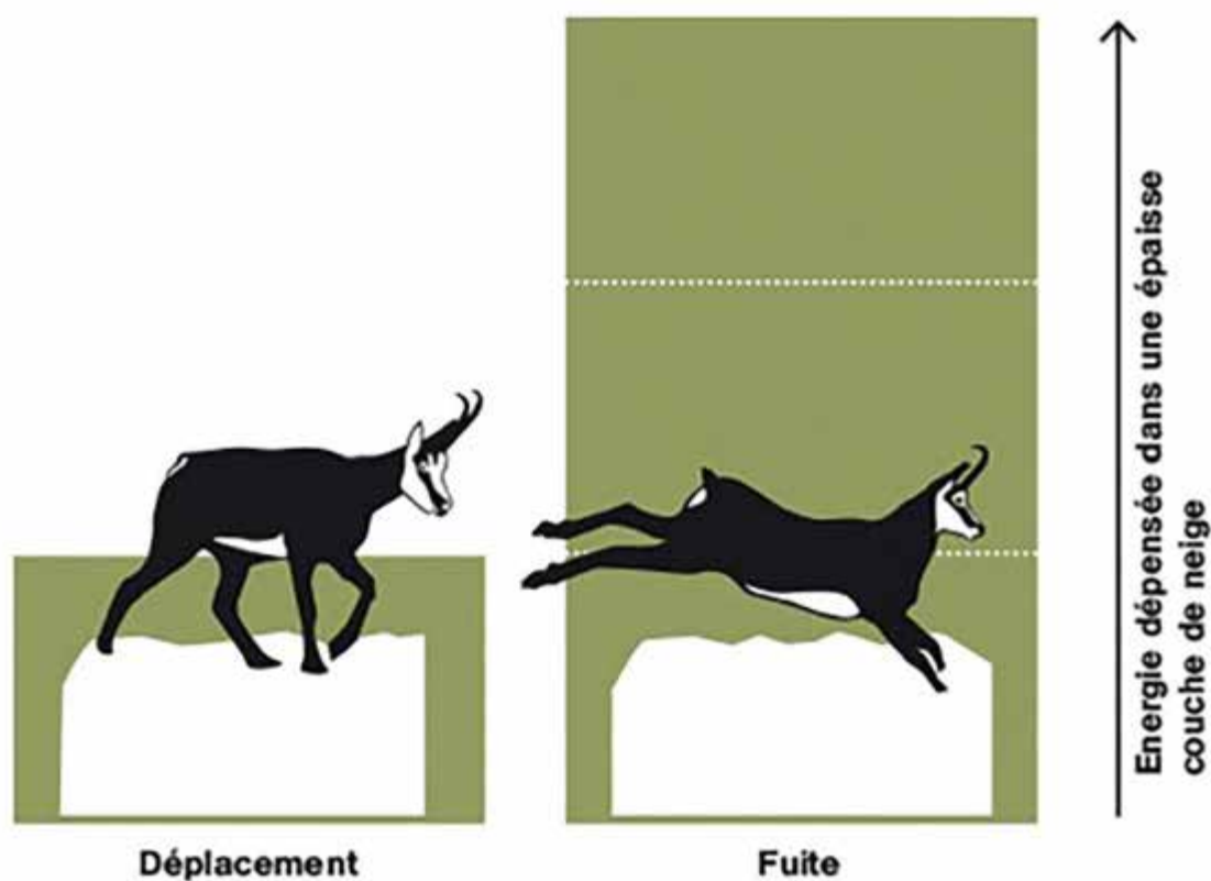
Figure 1 : Diagramme de l'énergie dépensée dans une épaisse couche de neige, tiré de l'association « Nature & Loisirs, connaître la faune ».
